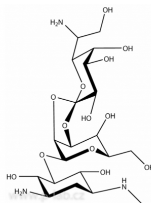
HYGROMYCIN B vzorec
