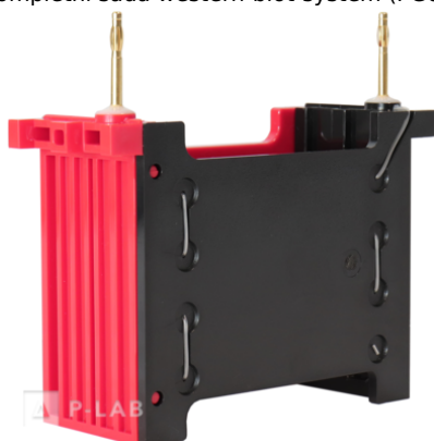
Rám s elektrodami
