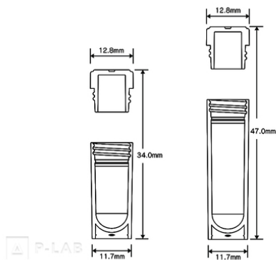
Kryozkumavky FastGene s vnitřním šroubovacím uzávěrem - technický náčrtek s rozměry
