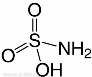
KYSELINA SULFAMOVÁ
