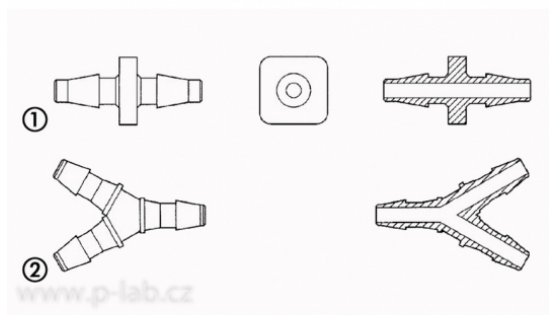
Spojka (1) a rozdvojka Y (2)
