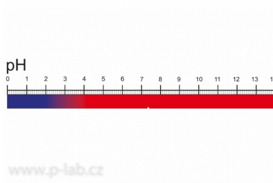
Barevný přechod pH indikátoru
