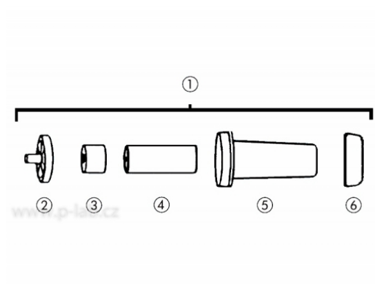
1 - Držák pipety - komplet
