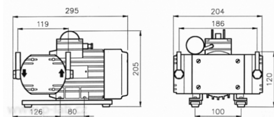
Schéma vývěvy 20D
