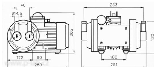
Schéma vývěvy 40D
