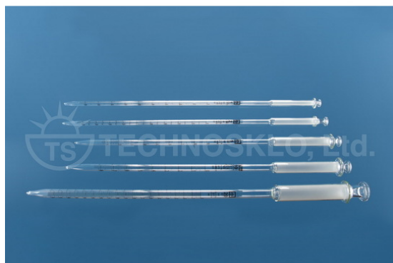
Pipeta dělená třída AS s pístem
