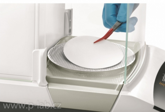
Semimikrováha Secura®
